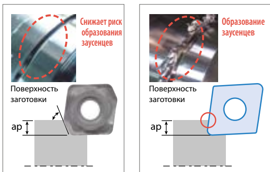
Стружколом SX
